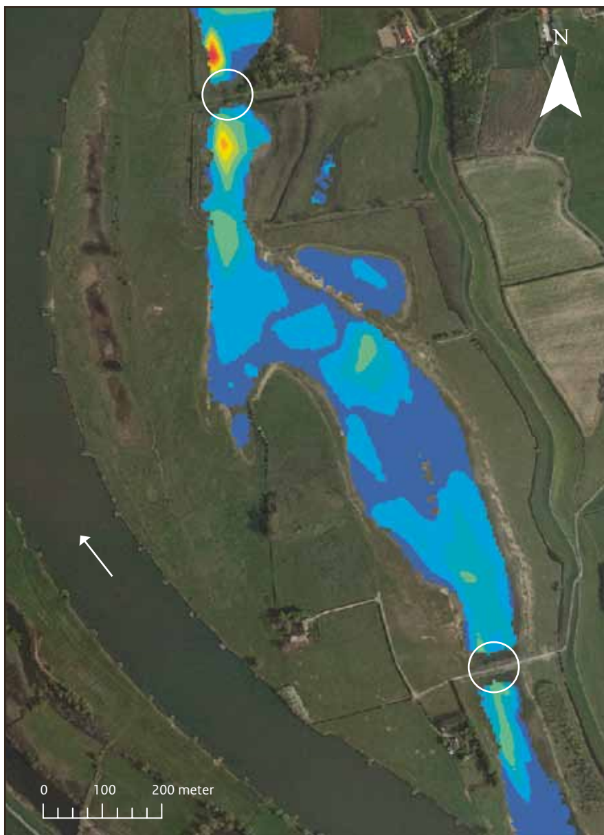
Figuur 16 Stroomsnelheden in de nevengeulen van de Vreugderijkerwaard op basis van een representatieve voorjaarsafvoer (2650 m 3 /s bij Lobith). De cirkels geven de regelwerken aan.
