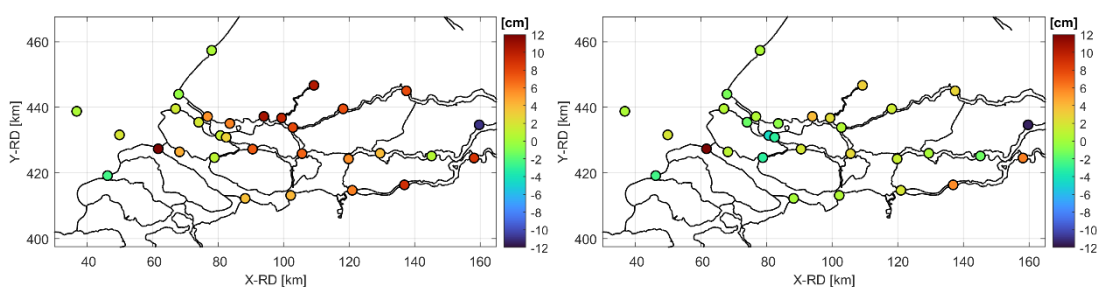
Figuur 2 Bias voor waterstanden van voor de kalibratie (links) en na kalibratie met OpenDA (rechts)
