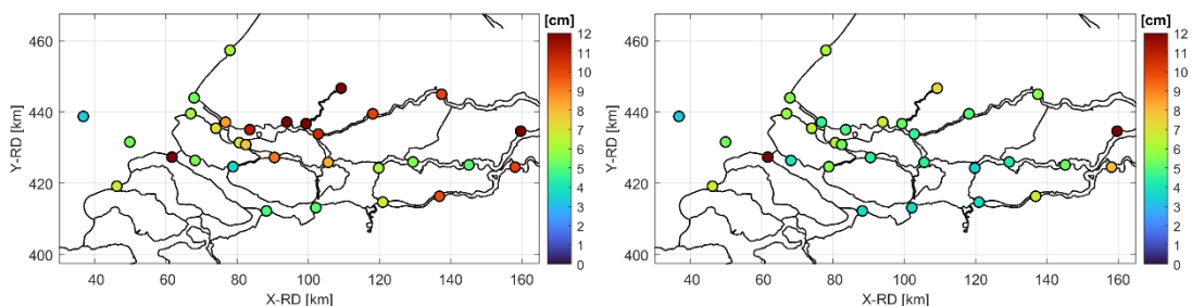
Figuur 3 RMSE voor waterstanden van voor de kalibratie (links) en na kalibratie met OpenDA (rechts)
