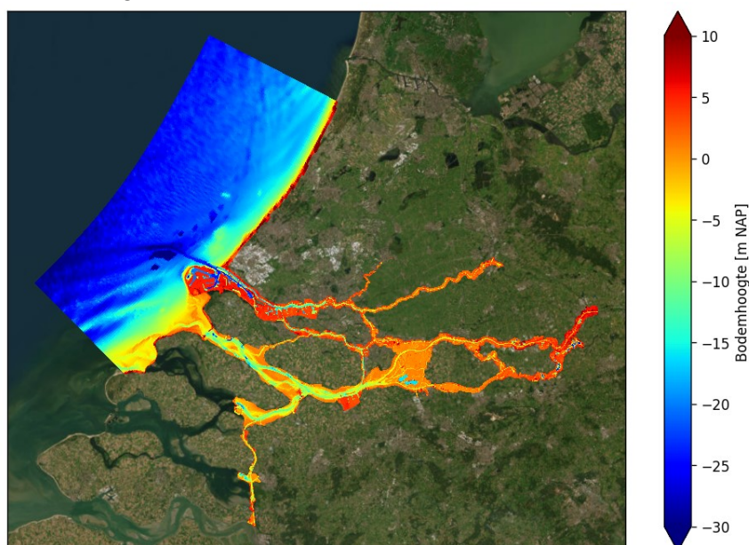
Figuur 1 Modelbodemoogte (D-HYDRO) van het volledige modelnetwerk
