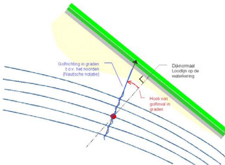
Figuur 3.4 Schematische weergave van de dijknormaal (in graden t.o.v. noord), golfrichting en hoek van golfval, uit Ministerie van Verkeer en Waterstaat (2007). In dit voorbeeld is de oriëntatie van de dijknormaal 225 ( ^{\circ} N) en de golfrichting in de rode stip 200 ( ^{\circ} N), de hoek van golfval is 25 graden.
