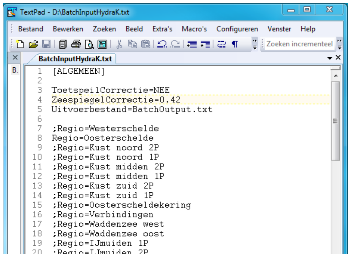
Figuur 2.2 Screenshot van een Hydra-K invoerbestand.
