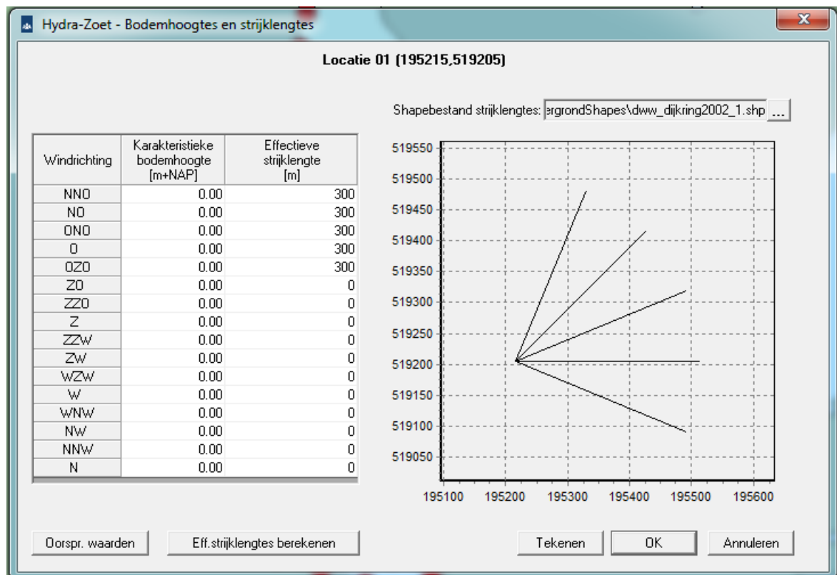
Figuur D.1 Screenshot van het invoerscherm 'Bodemhoogtes en strijklengtes' in Hydra-Zoet.
