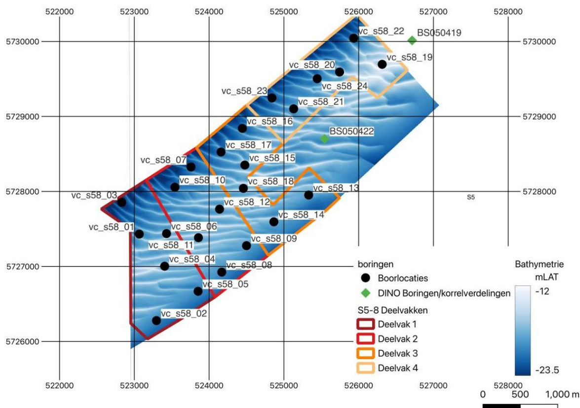
Figuur 4-3 Bodemhoogte van zandwinvak S50 (i.e. MER-vak S5-8) in 2022 en locatie van boringen met korrelgrootteverdelingen. Figuur overgenomen uit de gebiedsrapportage (Wiertsema & Partners, 2023).
