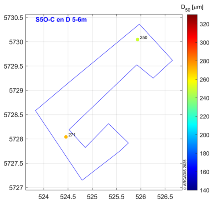
Figuur 4 Ruimtelijke variatie in D_{50} op een diepte van 5-6 m onder de zeebodem in zandwinvak S5O deelgebied 3 (C) en 4 (D).
