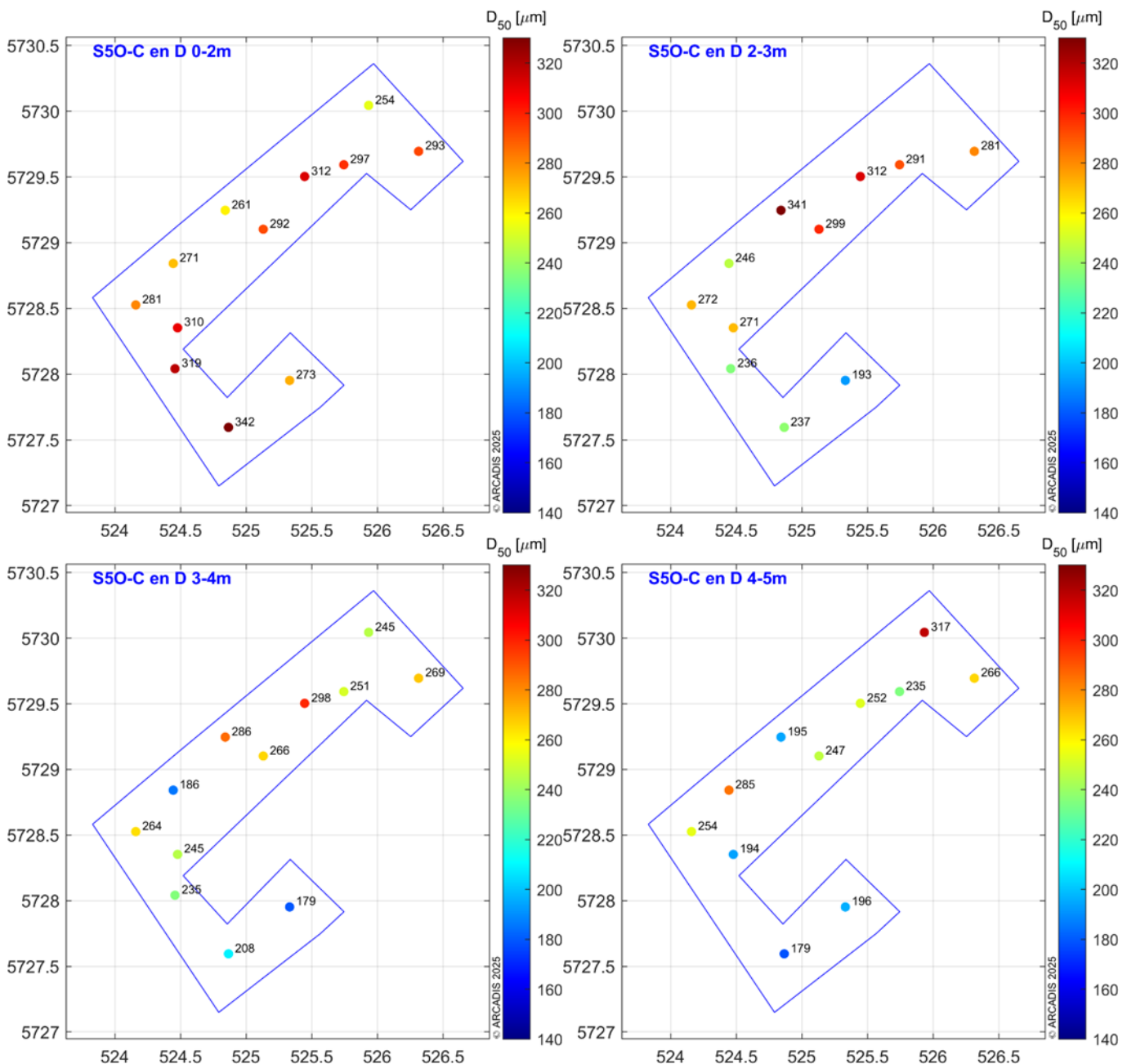
Figuur 3 Ruimtelijke variatie in D_{50} op een diepte van 0-2 m, 2-3 m, 3-4 m en 4-5 m onder de zeebodem in zandwink S50 deelgebied 3 (C) en 4 (D).
