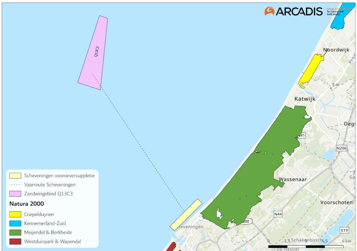
Figuur 1 Overzichtkaart van zandwinkvak Q13C3 (roze), het suppletievak inclusief uitloopraaien (geel) en de vaarroute daartussen ten opzichte van Natura 2000-gebied Coepelduynen, Kennemerland-Zuid, Meijendel & Berkheide en Westduinpark & Wapendal.
