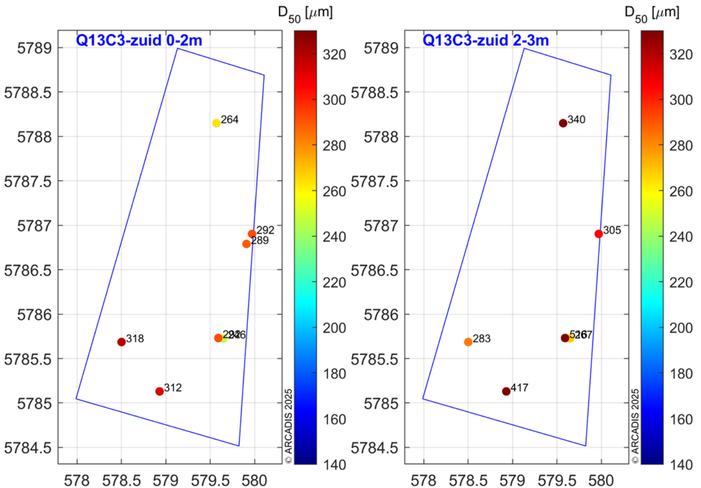
Figuur B4-1 Ruimtelijke variatie in D_{50} op een diepte van 0-2 m en 2-3 m -zb in zandwinkvak Q13C3-Zuid.
