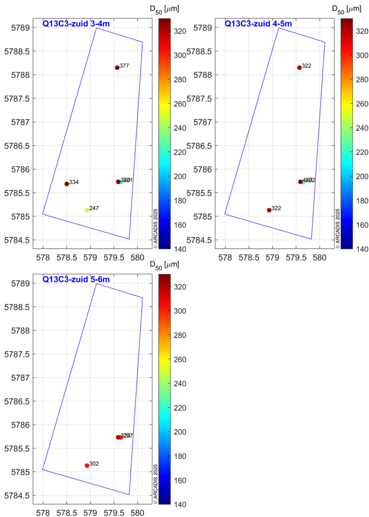
Figuur B4-2 Ruimtelijke variatie in D_{50} op een diepte van 3-4 m, 4-5 m en 5-6 m -zb in zandwinvak Q13C3-Zuid.
