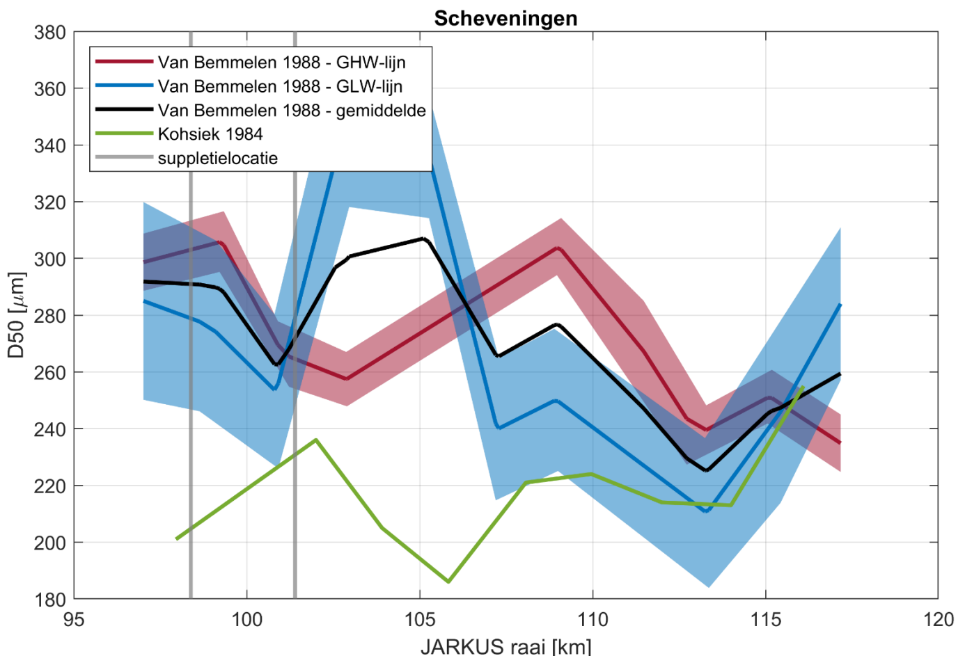
Figuur 4-2. D_{50} -waarden van Delfland uit de dataset van Van Bemmelen (1988) en Kohsiek (1984). De gemiddelde D_{50} -waarde van Van Bemmelen is berekend door het lopend gemiddelde van de GHW-lijn en de GLW-lijn te nemen. De grijze verticale lijnen tonen de suppletielocatie Scheveningen inclusief de uitloopraaien.
