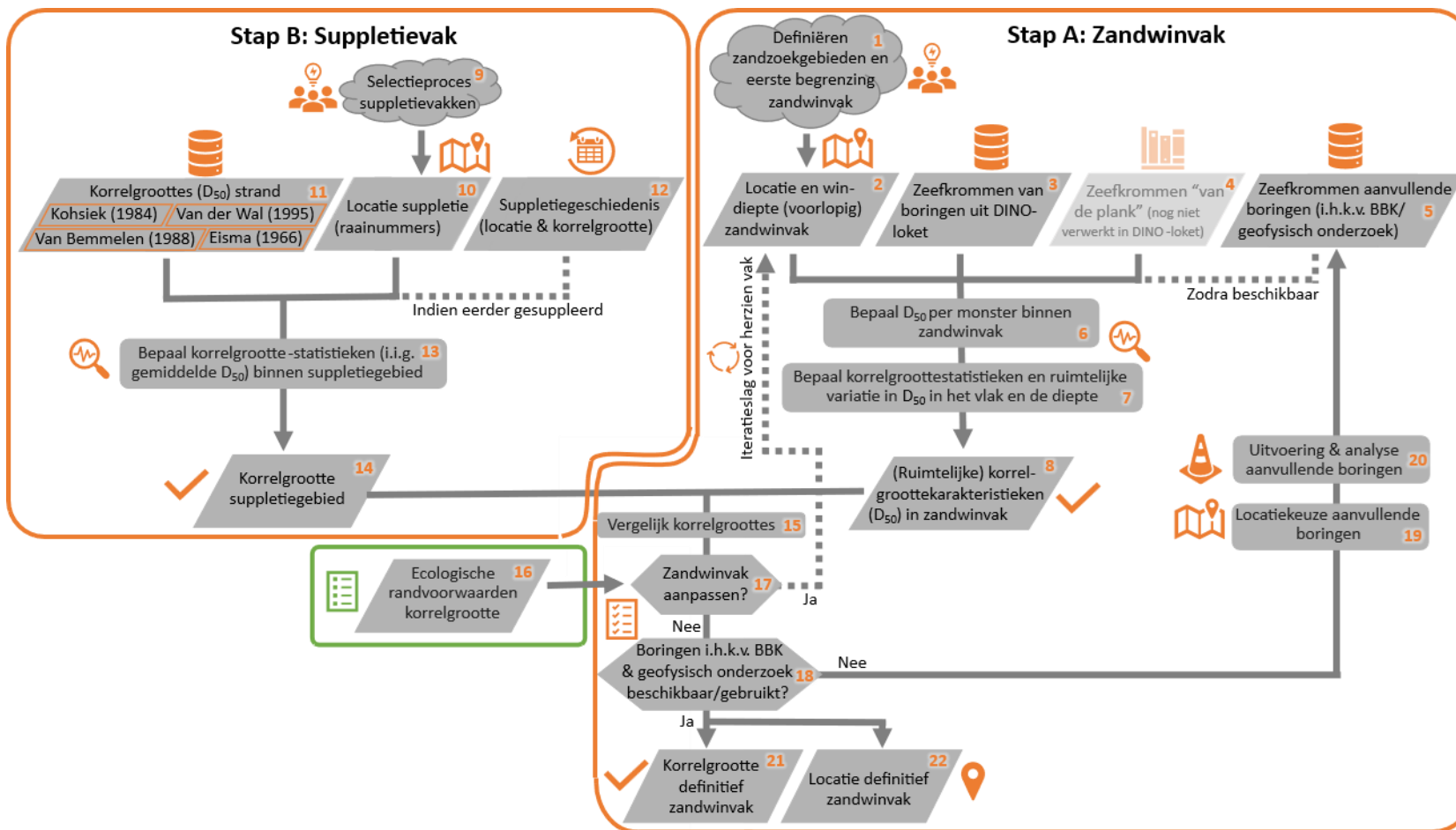
Figuur B1-0-1 Workflow voor bepalen en vergelijken van de korrelgrootte in een suppletievak en bijbehorend zandwinkvak.
