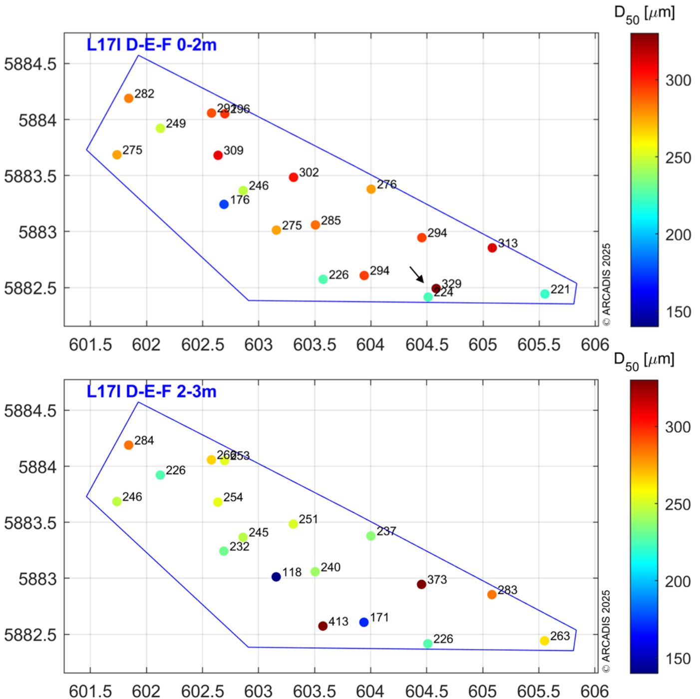
Figuur B4-1. Ruimtelijke variatie in D_{50} op een diepte van 0-2 m en 2-3 m -zb in zandwinkvak L17I deelvak D-E-F. De boring aangeduid met de pijl is de boring van vóór 2016. De rest van de boringen zijn allemaal genomen in 2021.
