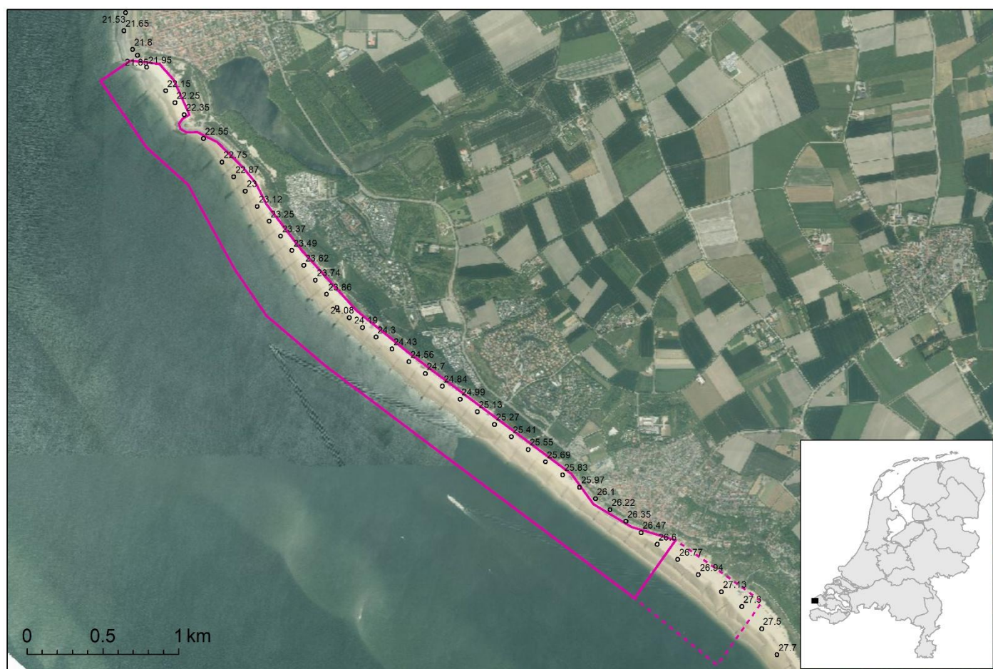
Figuur 4-1 Luchtfoto van de suppletielocatie uit 2023. De roze polygoon toont de raai begrenzing van het suppletievak inclusief uitloopraaien (stippellijnen).
