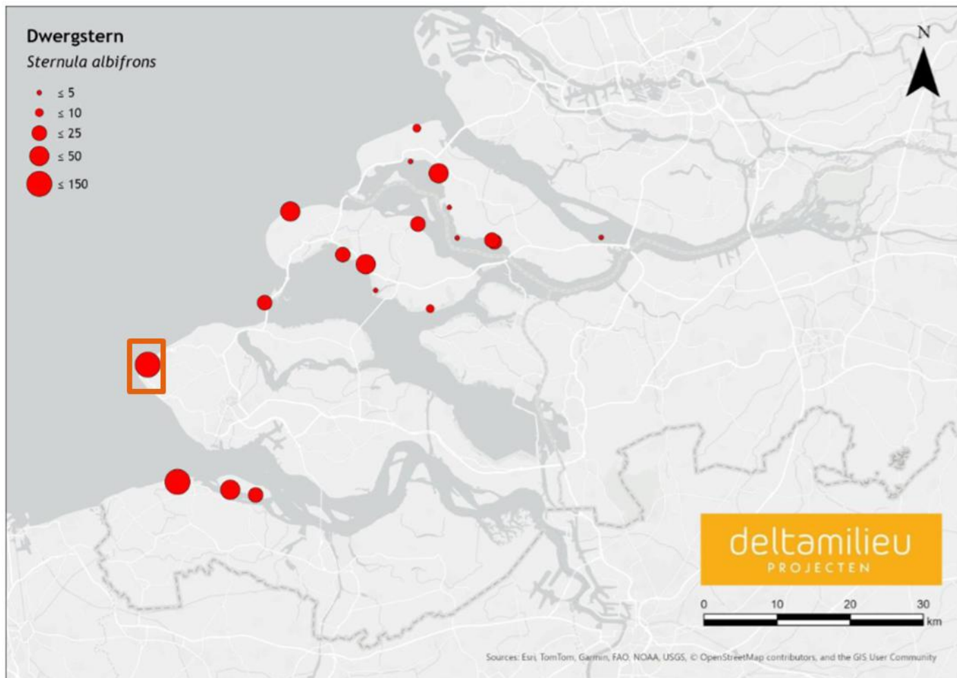
Figuur 3-4 Verspreiding van de dwergstern. Het oranje kader geeft het projectgebied aan (aangepast uit Lilipaly & Sluijter, 2025).
