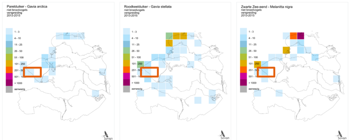
Figuur 4-1 Verspreiding van parelduikers (links), roodkeelduikers (midden) en zwarte zee-eend in Zeeland in de winter (periode 2013 tot 2015) (Sovon Vogelonderzoek Nederland, 2025b, 2025a). Het projectgebied is aangegeven met het oranje kader.
