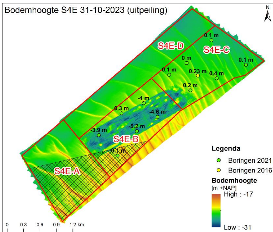
Figuur 4-3 Bathymetrie van zandwinnak S4E van 31-10-2023 (uitpeiling) na zandwinning, met de locatie van de boringen uit 2016 en 2021. Bij elke boring is de bodemhoogteverandering tussen het moment waarop de boring gezet is en de uitpeiling weergegeven; negatieve waarden duiden op zandwinning. De geruite driehoek in het zuiden is uitgesloten voor zandwinning. NB: de bodemhoogte t.o.v. LAT is hier gelijk aan de bodemhoogte t.o.v. NAP plus ca. 1,9 m (Ministerie van Defensie, 2020).
