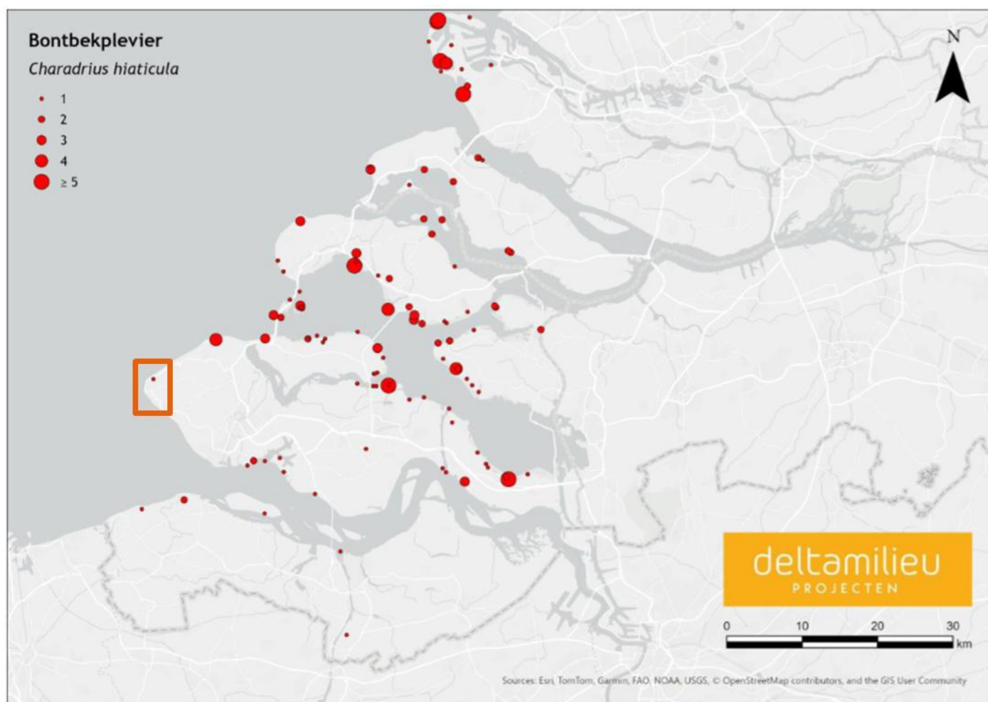
Figuur 3-3 Verspreiding van de bontbekplevier in het Deltagebied. Het oranje kader geeft het projectgebied aan (aangepast uit Lilipaly & Sluijter, 2025).
