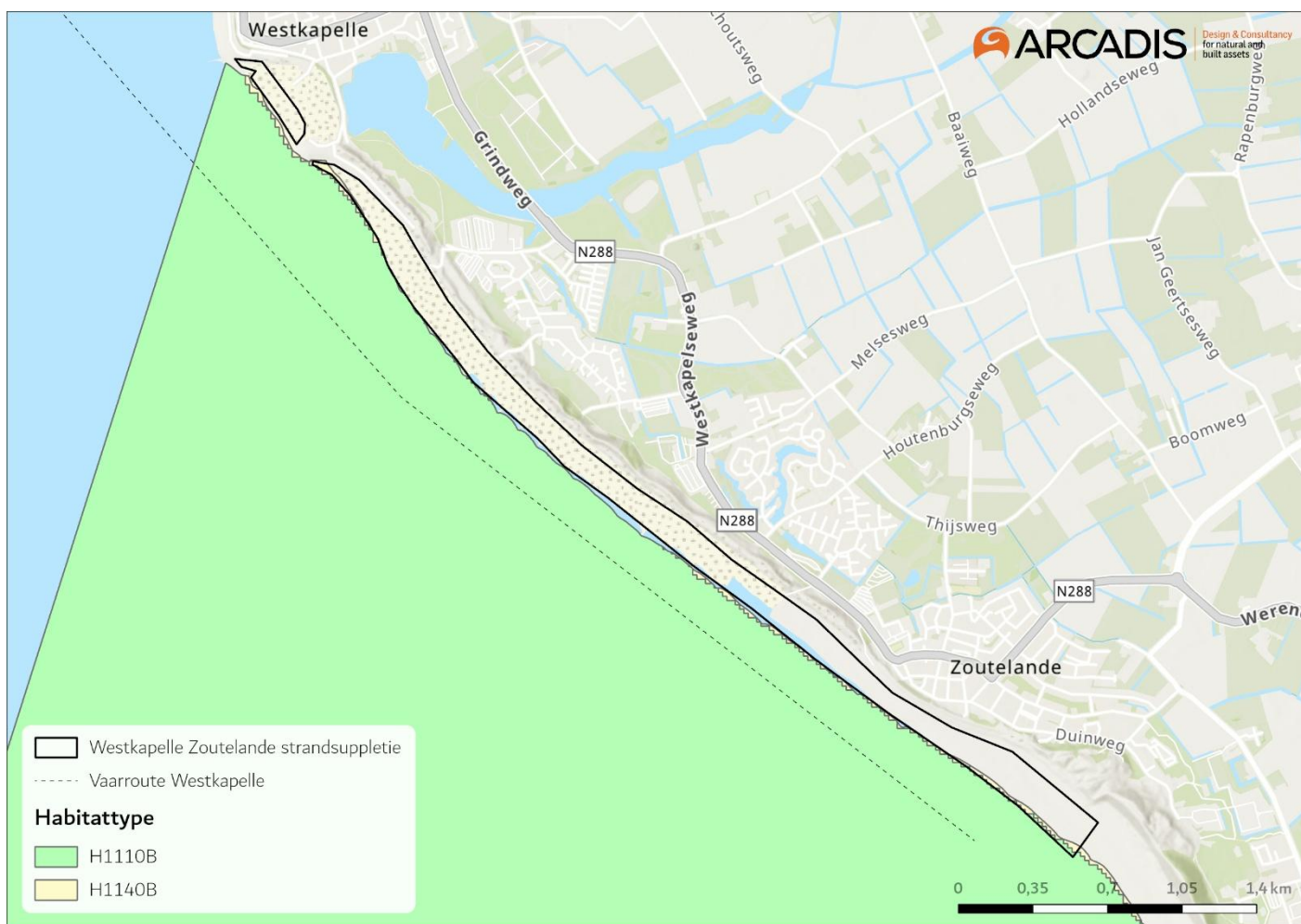
Figuur 3-5 Habitattypen in de Westerschelde. Er liggen geen gevoelige duintypen nabij de suppletielocatie.
