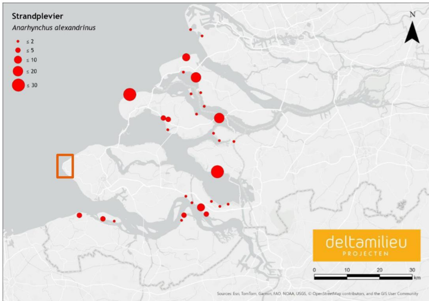
Figuur 3-2 Verspreiding van de strandplevier. Het oranje kader geeft het projectgebied aan (aangepast uit Lilipaly & Sluijter, 2025).
