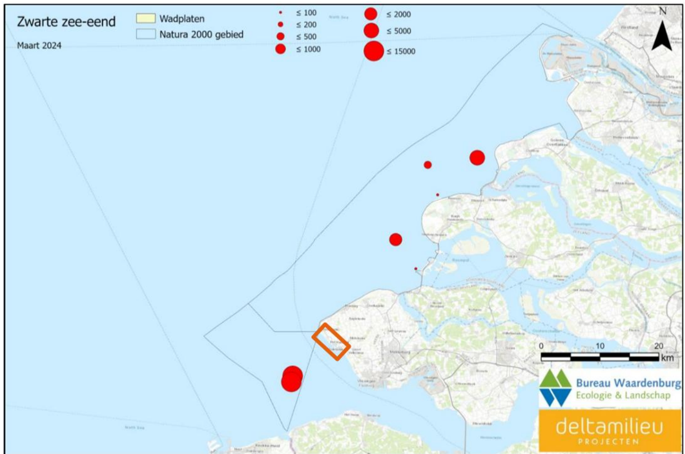
Figuur 4-2 Verspreiding van Zwarte zee-eenden in de Voordelta in maart (Sluijter & Wolf, 2024)). Het projectgebied is aangegeven met het oranje kader.
