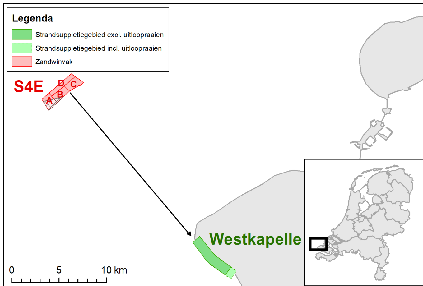
Figuur 2-1 Overzicht van de ligging van het suppletiegebied Westkapelle (groen) en het voorgenomen zandwinvak (rood). Alleen deelvak B en C van het zandwinvak worden voor deze suppletie gebruikt. Het grijs geruite deel van het zandwinvak is uitgesloten voor zandwinning. Gestippelde deel van het suppletiegebied betreft de uitloopraaien.
