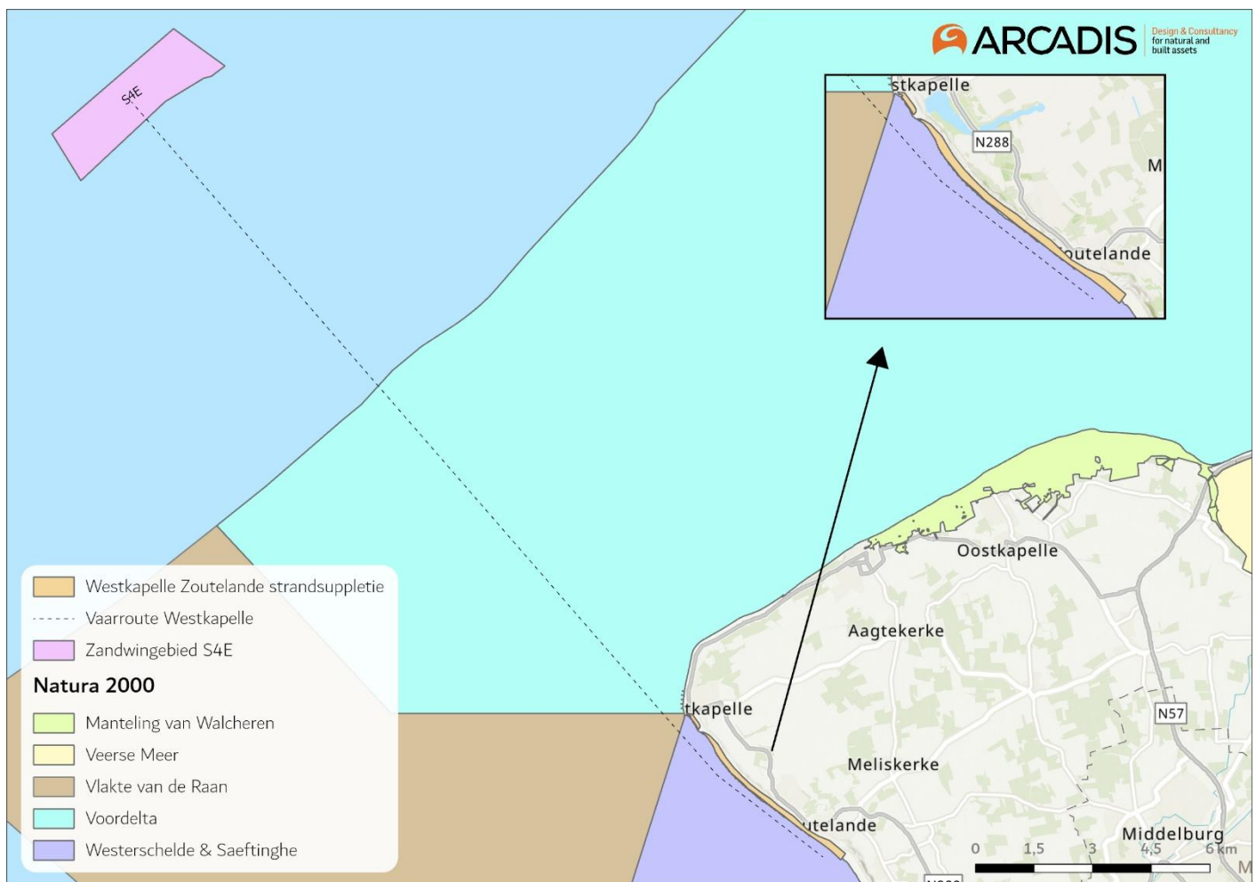
Figuur 2-1 Overzichtskartaal van zandwinkvak S4E (roze), de suppletievak inclusief uitlooppraaien (oranje) en de vaarroute daartussen ten opzichte van Natura 2000-gebieden Voordelta, Vlakte van de Raan en Westerschelde.
