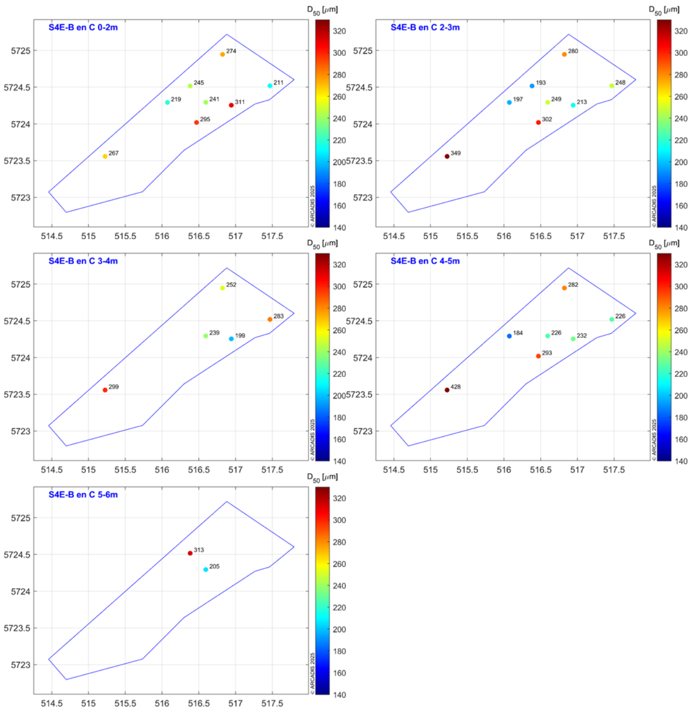
Figuur B4-1. Ruimtelijke variatie in D_{50} op een diepte van 0-2 m, 2-3 m, 3-4 m, 4-5 m en 5-6 m -zb in zandwinkvak S4E deelvak B en C.
