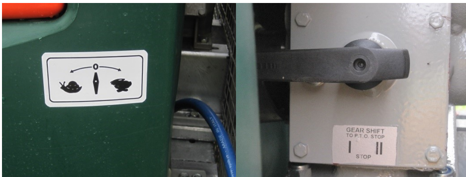
Figuur 5 Stand van de overbrengingsverhouding van de aftakas op de ventilator op de Lochmann NL dwarsstroomspruit met ACS (links: indicatie op de spuittank en rechts: stand van de tandwielkast met behulp van een handgreep (hendel)).
