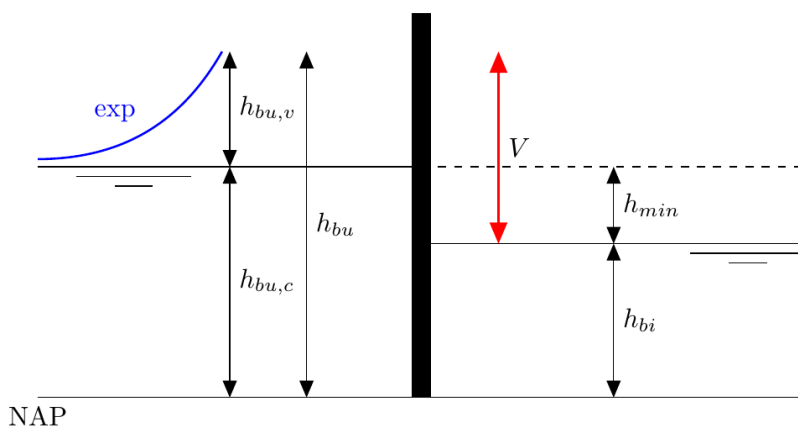
Figuur 4 – Situatieschets
