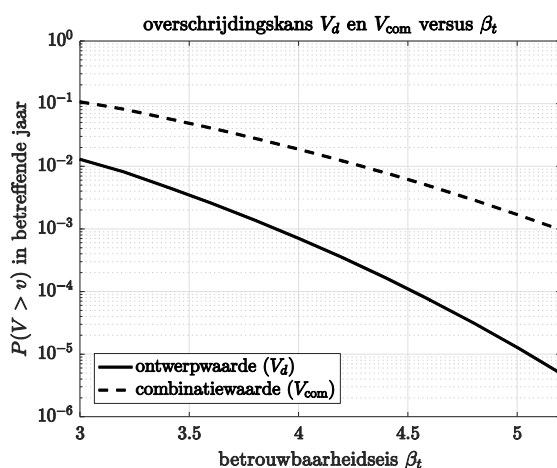
Figuur 19 – Ontwerpwaarde en combinatie waarde van de vervalbelasting voor toetsing van het eerste of laatste levensjaar (y-as) als functie van de betrouwbaarheidseis (x-as), uitgedrukt in de kans van overschrijden in het betreffende levensjaar
