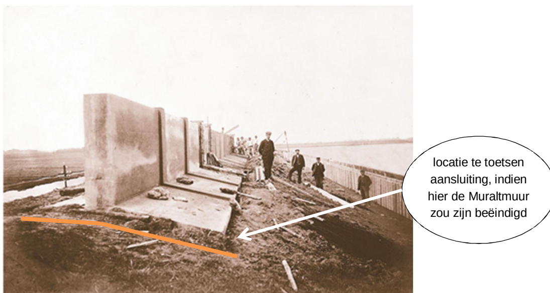
Figuur 2-10: Voorbeeld van loodrechte aansluiting boven kruin uitstekende wandconstructie (#26), foto van werk aan fundering van Muralmuur op Schouwen-Duiveland 1903-1908 (bron: www.zeeuwseankers.nl )
