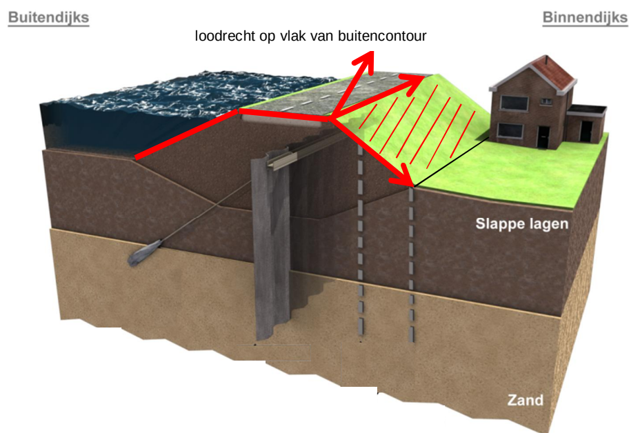
Figuur 2-2: Toelichting op het vlak van de buitencontour van waterkering
