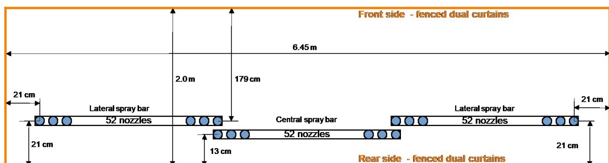
Figuur 2: Afmetingen van ARA600
