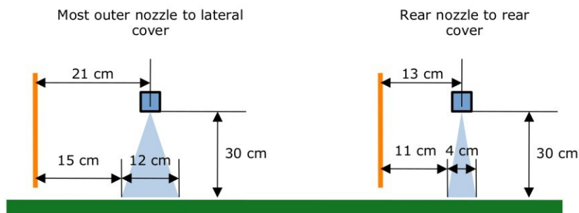
Figuur 3: Positie van de buitenste spuitdop ten opzichte van de zijdelingse afdekking met aanduiding van de spuitbreedte van de dop (links). Positie van de achterste spuitdop van de centrale spuitboom ten opzichte van de achteroverkapping met aanduiding van de verspoten lengte in de rijrichting (rechts).
