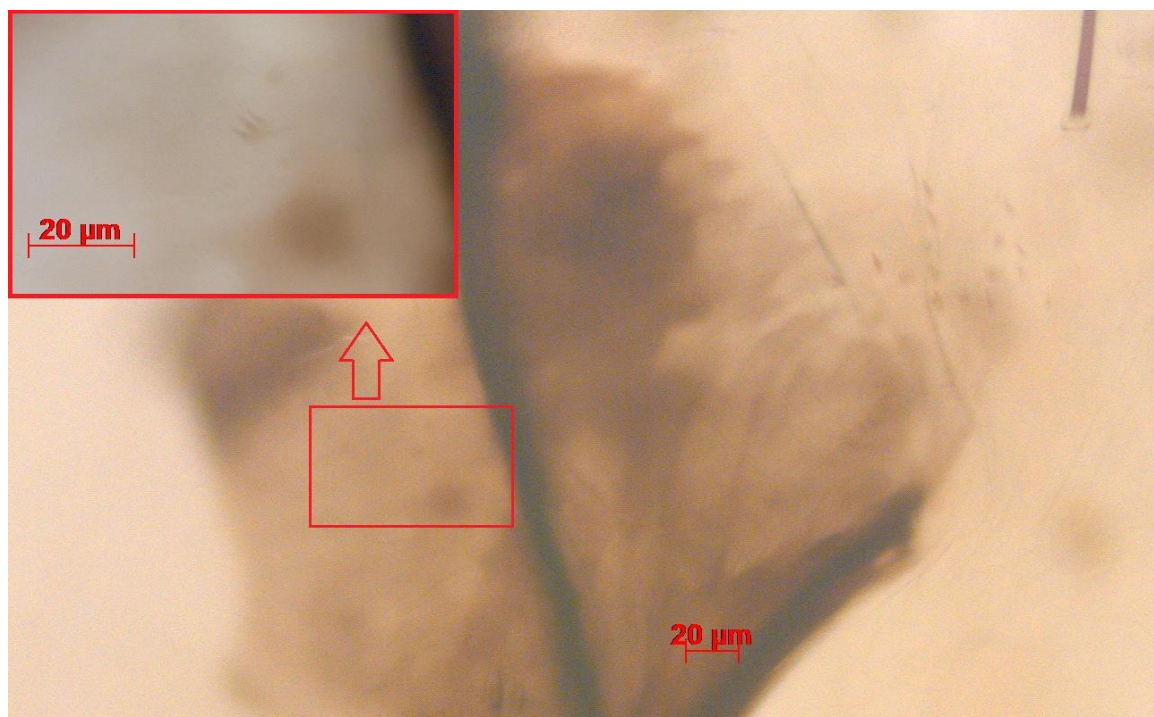
Foto 6 Coxopleuriet Mystacides , onderste helft relatief weinig stekelkammetjes en bovenste helft met één nauwelijks zichtbaar stekelkammetje.
