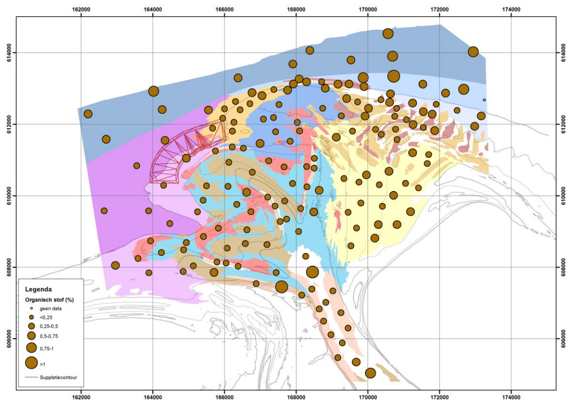
Figuur 4-3: % organisch stof in het Amelandse zeegat
