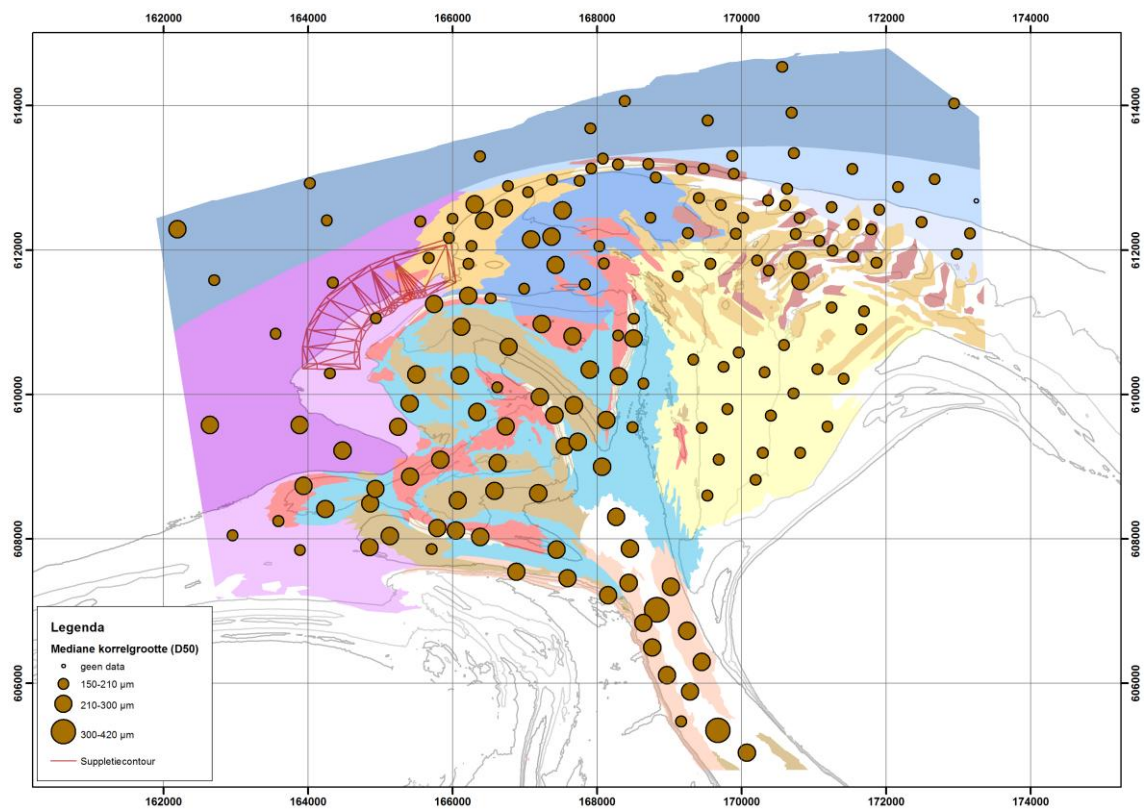
Figuur 4-2: Mediane korrelgrootte (D50) in het Amelandse zeegat
