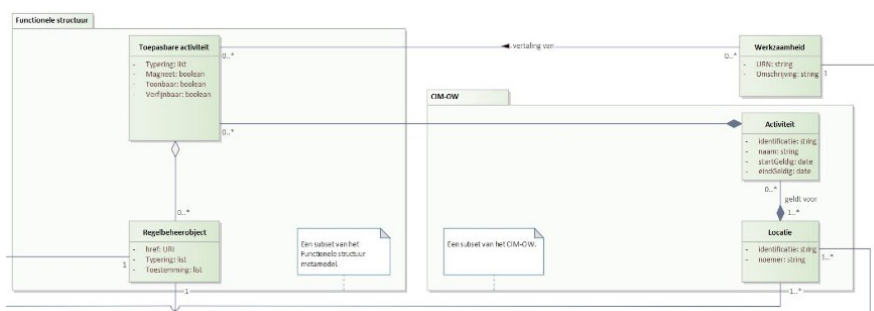
Figuur 17: Klassendiagram Informatiemodel Functionele Structuur
