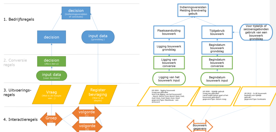
Figuur 2: IMTR lagen en DMN beslissstructuur
