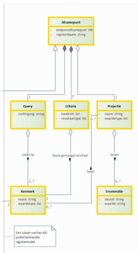
Figuur 16: Klassendiagram IMTR ExtensionElements API profiel gedeelte
