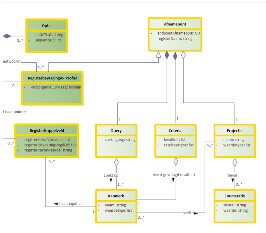
Figuur 9: Klassendiagram Registerbevraging API-profiel
