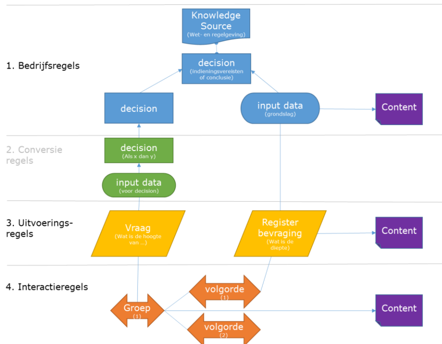
Figuur 1: Lagenmodel IMTR
