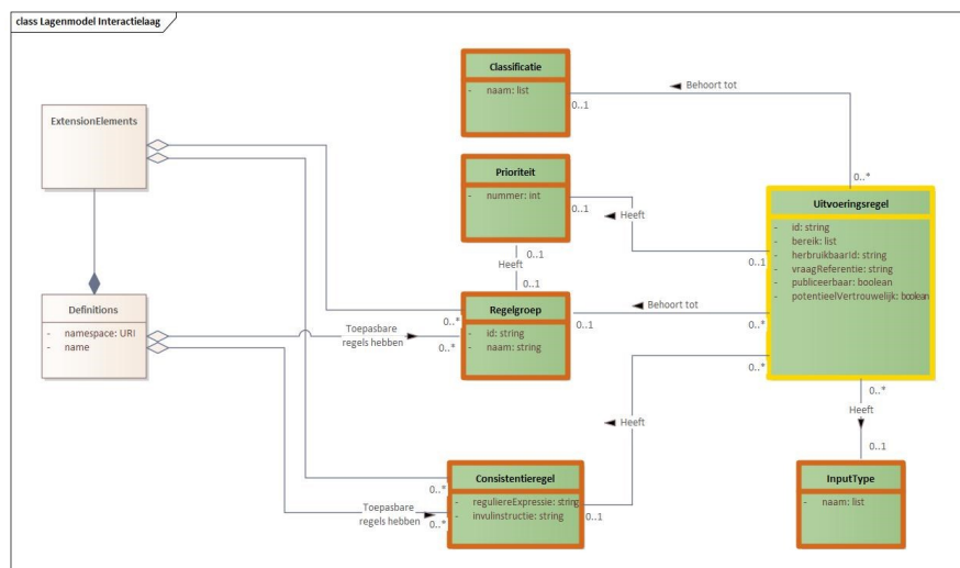
Figuur 11: Interactieregels waaraan de uitvoeringsregels zijn gekoppeld
