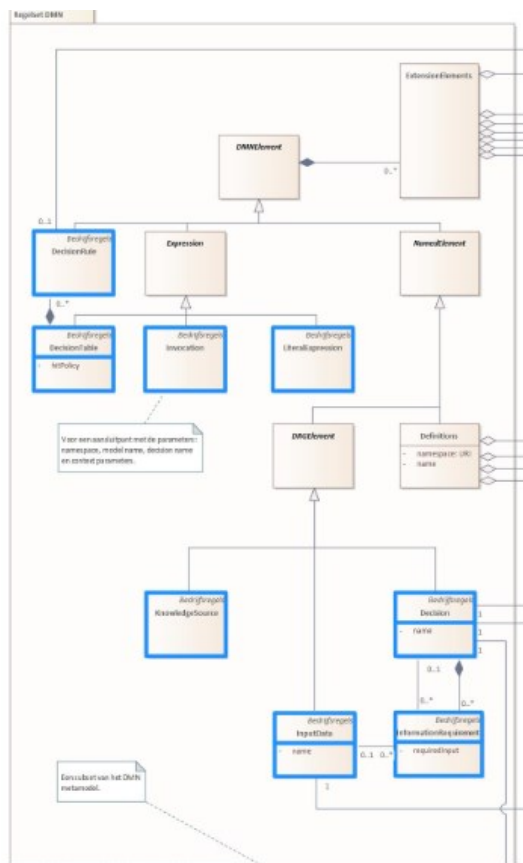
Figuur 14: Klassendiagram IMTR DMN gedeelte
