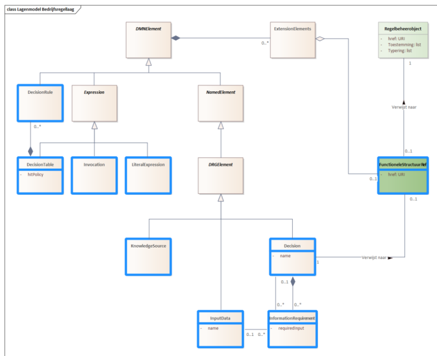
Figuur 4: Klassendiagram Bedrijfsregellaag
