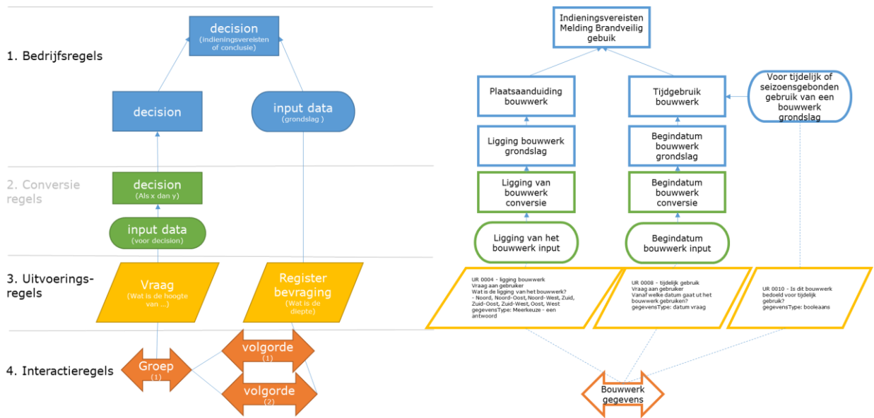
Figuur 2: IMTR lagen en DMN basisstructuur
