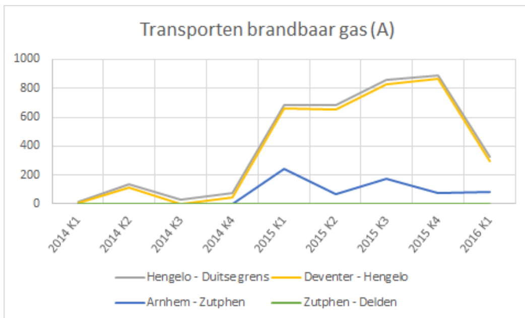
Figuur 13. Verloop transporten brandbare gassen tussen Arnhem, Deventer en Hengelo
