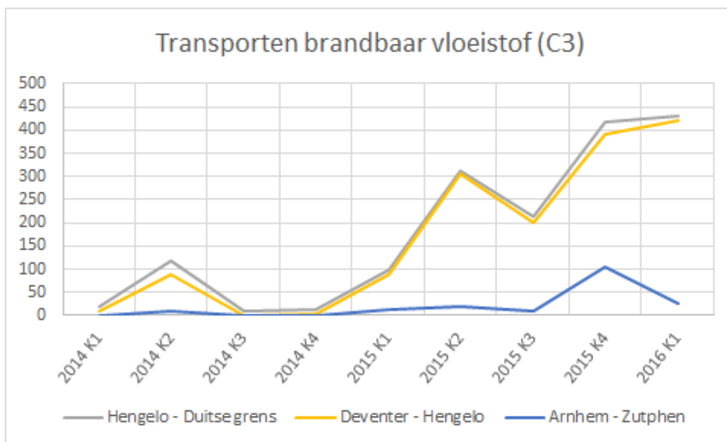
Figuur 14. Verloop transporten brandbare vloeistoffen tussen Deventer – Hengelo – Duitse grens
