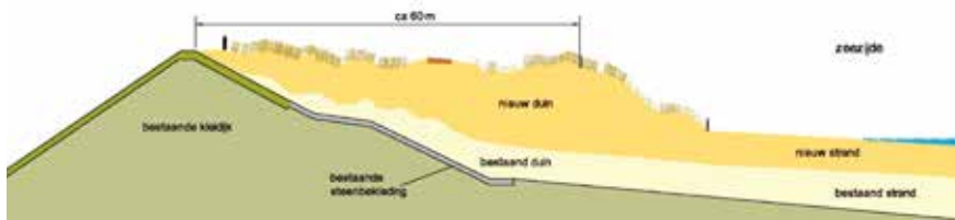
Figuur 9: Dwarsdoorsnede zandige versterking Nieuwvliet-Groede
