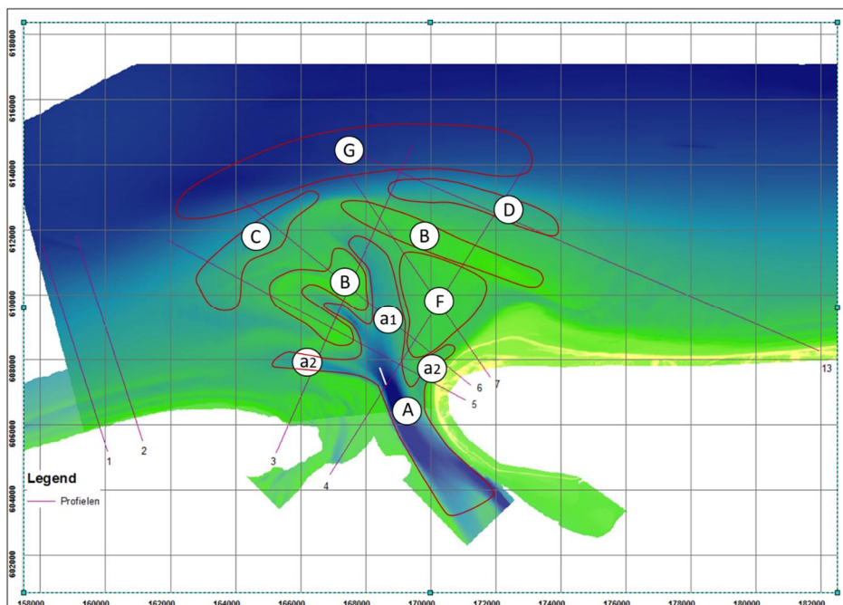
Figuur 2.2.3. Onderscheiden subgebieden op de buitendelta van het Amelander Zeegat op basis van een aantal gemeten en verwachte fysische kenmerken
