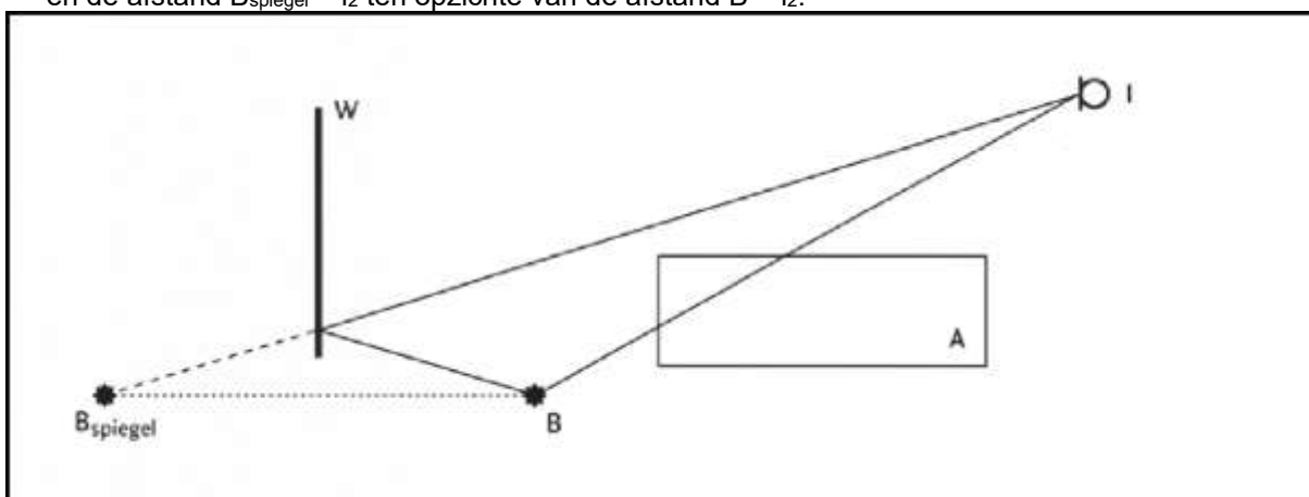
Figuur 3.3 Situatie met verschillende overdrachten
