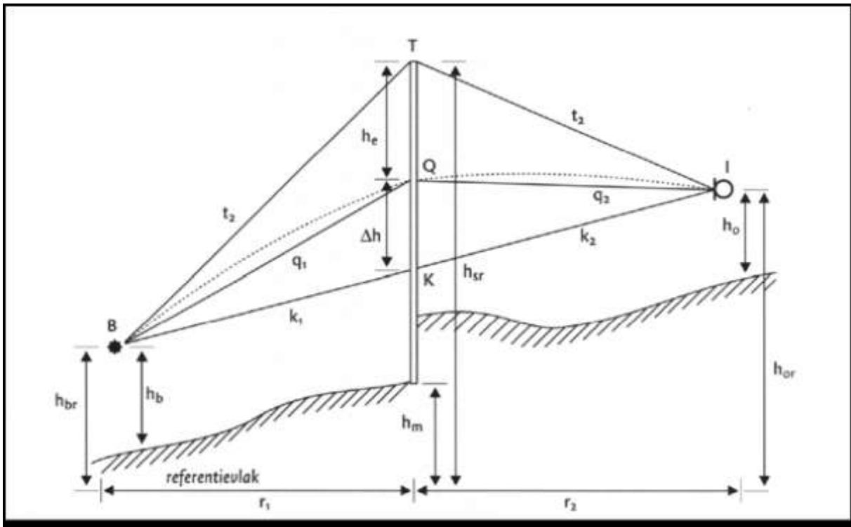
Figuur 3.5 Toelichting op de geometrische parameters bij de berekening van D_{\text{scherm}}
