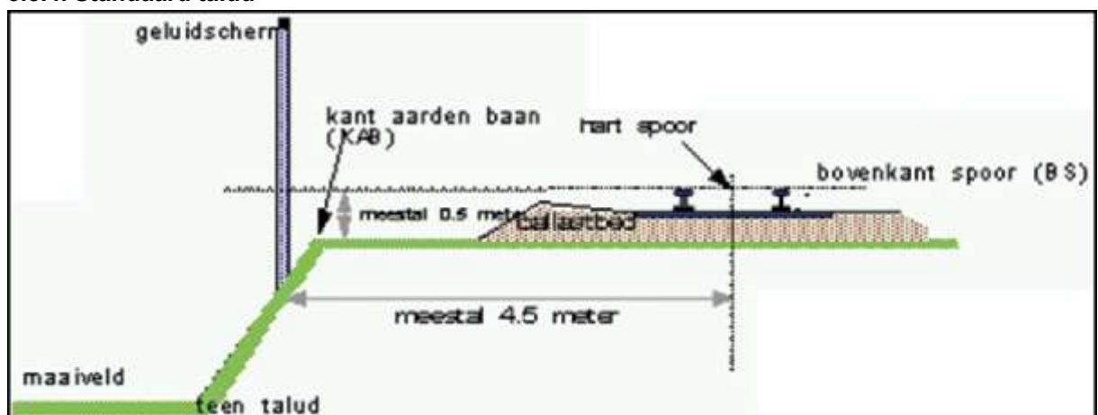
Figuur 3.2 Scherm op een verhoogde baan; het gemiddelde maaiveld links is wat lager dan de bovenzijde en rechts wat hoger dan naast het talud. De situatie rechts is bepalend voor h_T .
