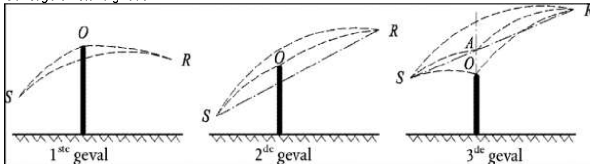
Figuur 2.5.e, Berekening van het padverschil in gunstige omstandigheden (enkele diffractie)
