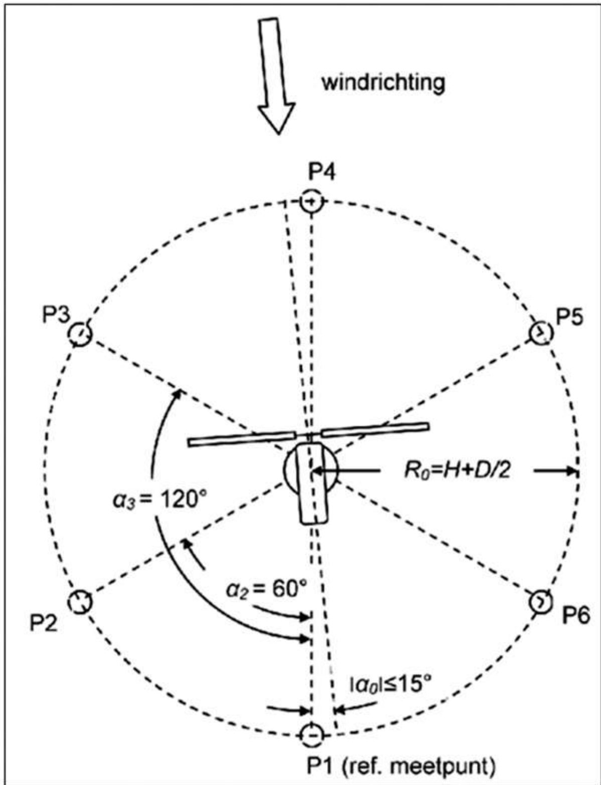
Figuur 1.1 bovenaanzicht van de geluidmeetposities
