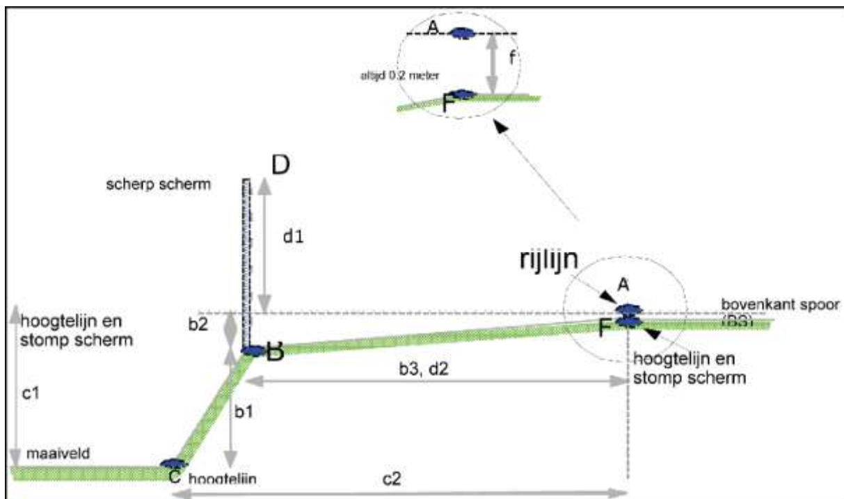
Figuur 3.4 Modellering van de dwarsdoorsnede van een standaard talud.
