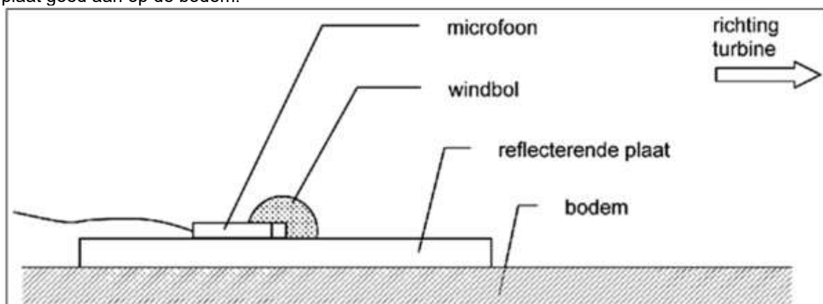
Figuur 1.3 weergave van de meetopstelling
