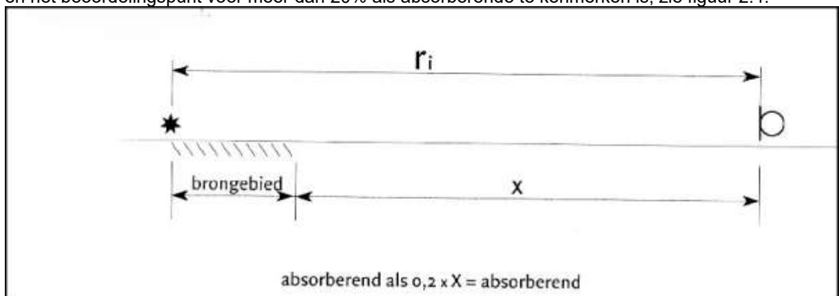
Figuur 2.4 Definitie absorberende bodem bij beoordelingspunt
