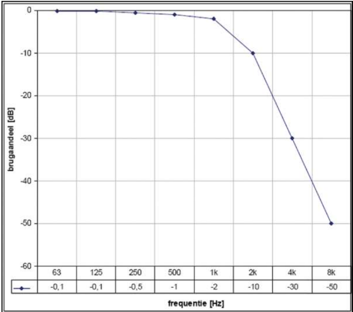
Figuur 4.2 Spectrale karakteristiek van het filter om het brugaandeel uit het verschilspectrum te filteren.
