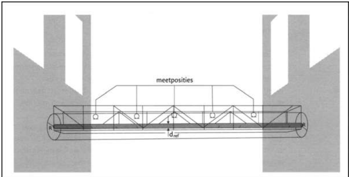
Figuur 2.12 Voorbeeld van een geluidvermogenmeting aan een compressorleiding (bevestigd aan een leidingbrug die als vakwerk licht is getekend)
