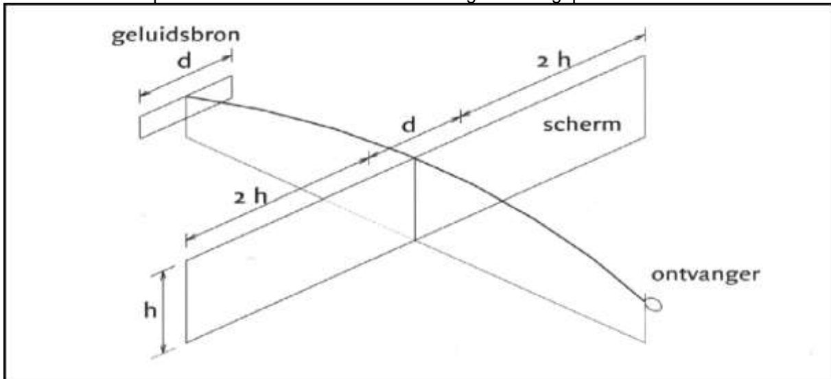
Figuur 3.1 Toelichting ruimtelijke specificatie verticale afschermingen
