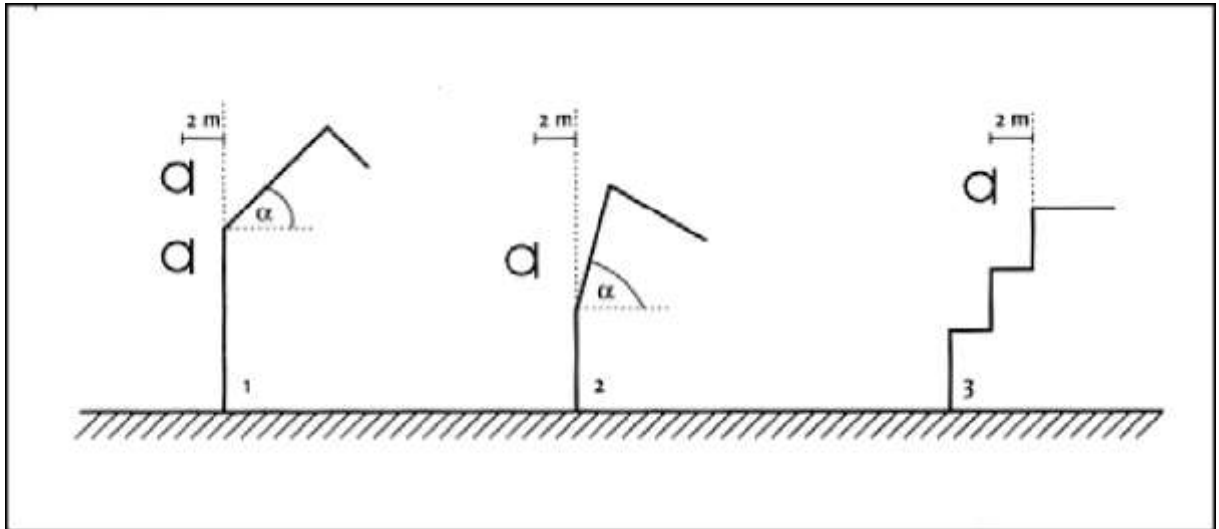
Figuur 4.2 Toelichting op gevelreflectie
