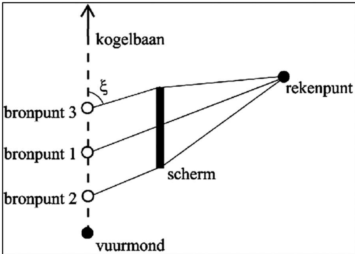
Figuur 4.12: Schematische weergave van afscherming van kogelgeluid.
