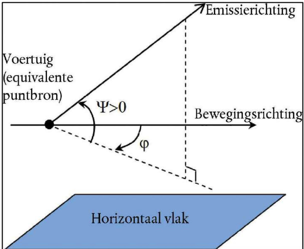
Figuur 2.3.b, Geometrische definitie
