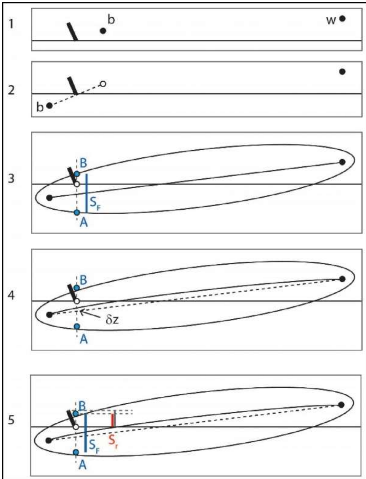
Figuur 3.6. Illustratie van vijf stappen (1-5) voor de berekening van SF en S_r , voor reflectie aan een hellend oppervlak.
