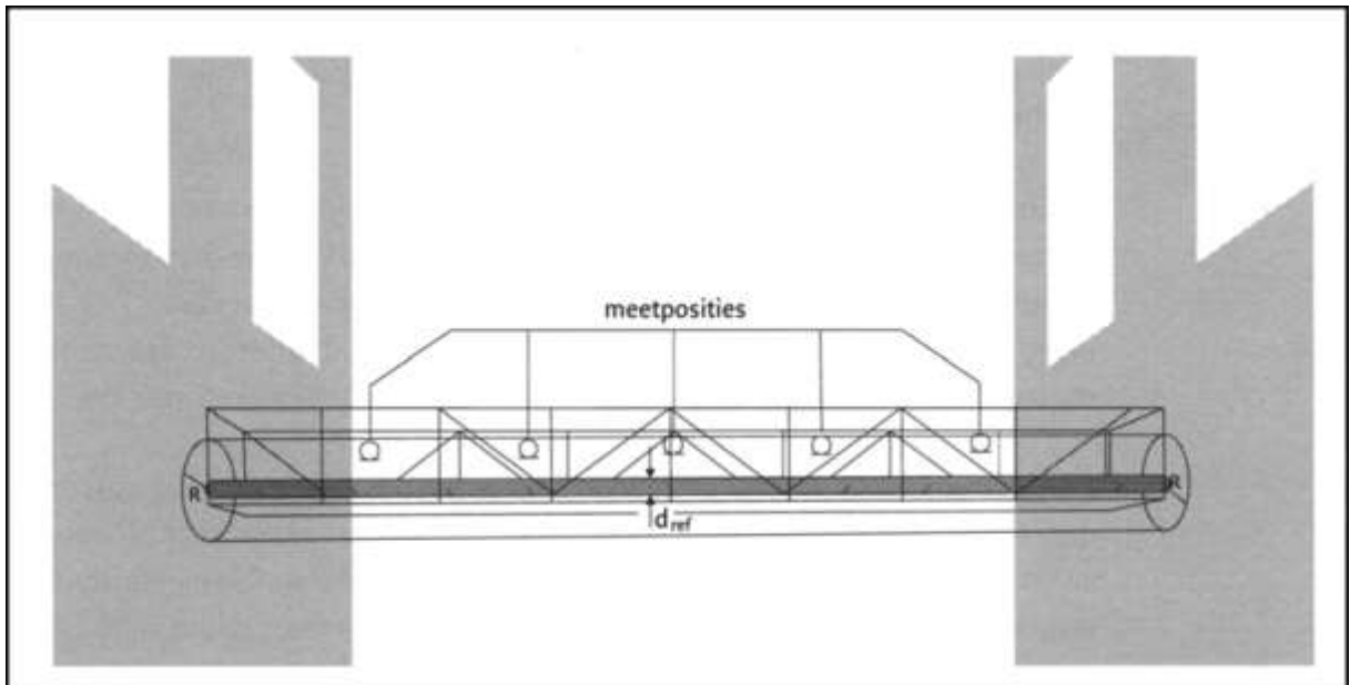
Figuur 2.8 Voorbeeld van een geluidvermogenmeting aan een compressorleiding (bevestigd aan een leidingbrug die als vakwerk licht is getekend)
