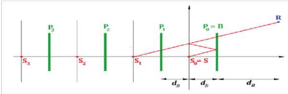
Figuur 2.5.k, Weergave van de modellering van meervoudige reflecties tussen trein en geluidscherm. Het geluidsvermogen van de equivalente bron wordt uitgedrukt door:
