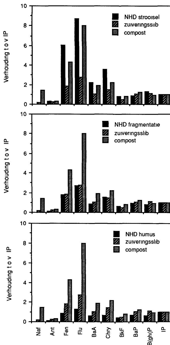
Figuur 3 PAK-profielen voor relatief schone organische toplagen in een bosbodem uit het Noordhollands Duinreservaat vergeleken met het profiel voor zuiveringsslib en compost. De hoeveelheid van iedere individuele PAK wordt uitgedrukt ten opzichte van de hoeveelheid indeno(1,2,3-cd)pyreen. Naf = naftaleen, Ant = antra-ceen, Fen = fenanteen, Flu = fluoranteen, BaA = benzo(a)antra-ceen, Chry = chryseen, BkF = benzo(k)fluoranteen, BaP = benzo(a)pyreen, B(ghi)P = benzo(ghi)perylene, IP = indeno(1,2,3-cd)pyreen. Naftaleen is niet gemeten in het NHD.
