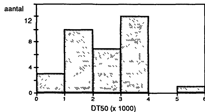
Figuur 1. Frequentieverdeling van de hoogte van DT50's voor een aantal microverontreinigingen. De DT50's zijn gebruikt om normen voor deze stoffen in zuiveringsslib en compost te berekenen (2)
