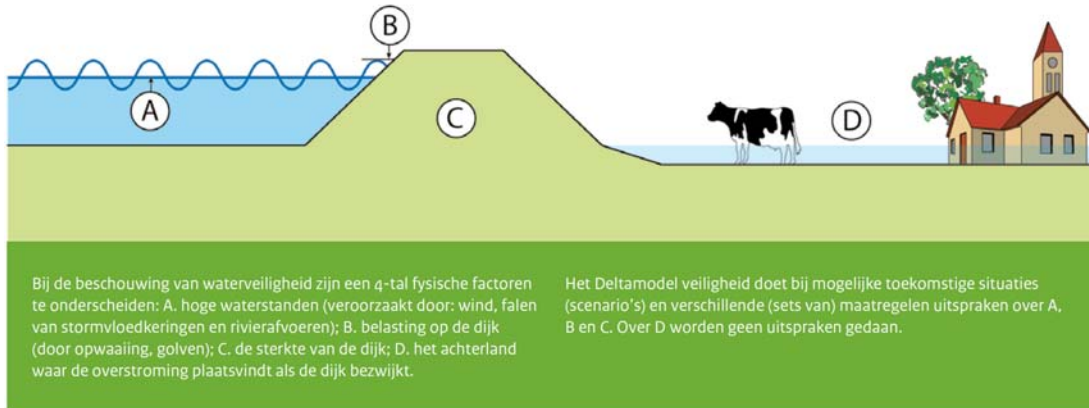
Figuur 4: Vier factoren die bij de beschouwing van de effecten op waterveiligheid te onderscheiden zijn
